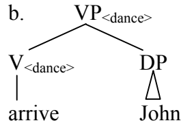
Unaccusative
